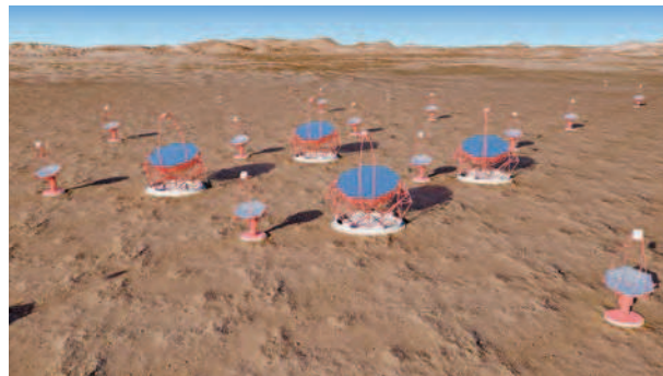
FIG. 5. Il progetto CTA (Cherenkov Telescope Array) per l'astronomia dei raggi gamma di alta energia.
